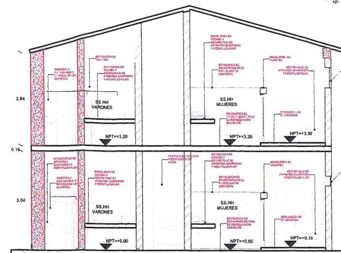
SECCIÓN C-C
