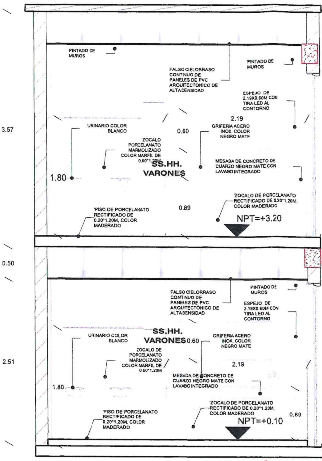
SECCIÓN A-A ESC: 1/50
