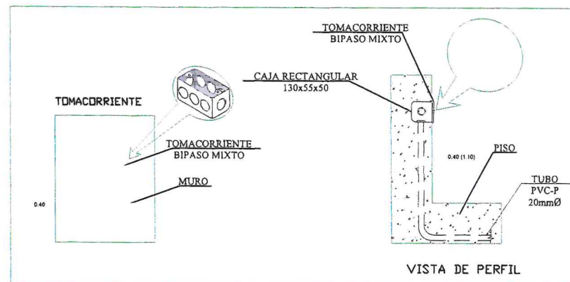
DETALLE: MONTAJE E INSTALACIÓN SALIDA DE TOMACORRIENTE DOBLE SCHUKO, EMPOTRADA EN MURO T.N. 0.40m ESC: 3/4
