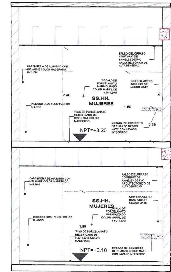
SECCIÓN A-A ESC: 1/50
