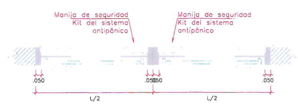
Planta esc. 1:25
