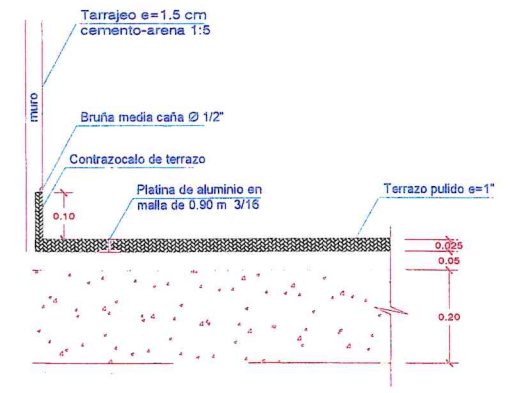
Detalle de piso de terrazo escala 1:10
