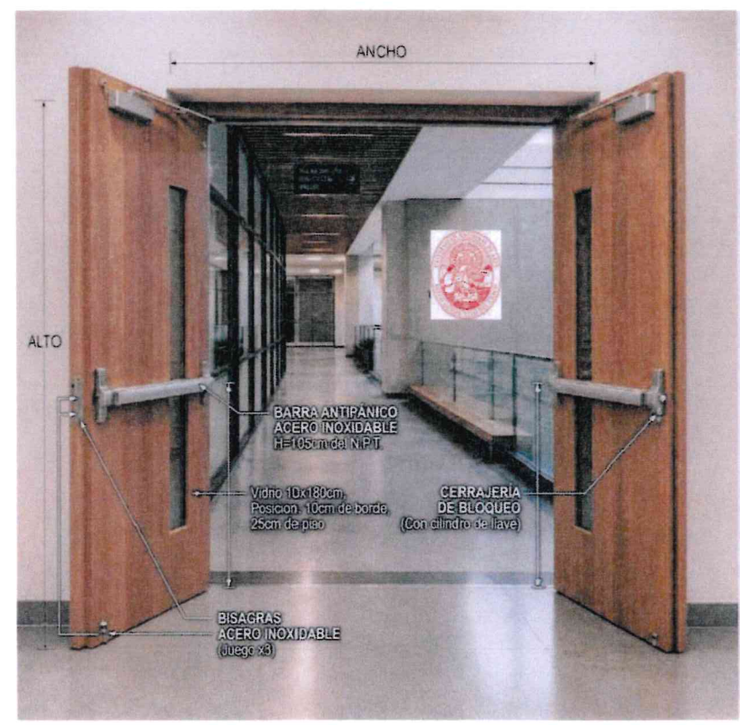
Elevacion Puerta Antipánico esc. 1:25
