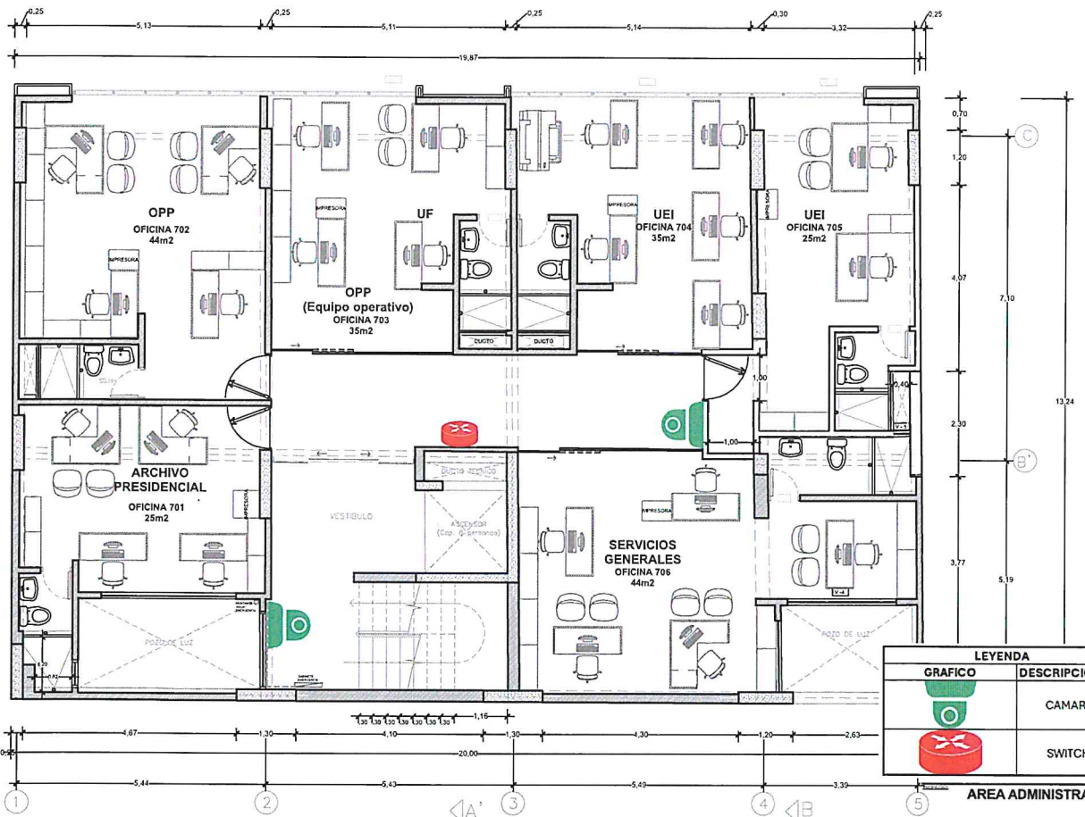
PLANO DE PLANTA 7mo NIVEL
